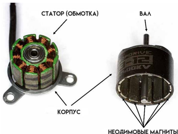
Рис. 60. Бесщёточный электродвигатель
