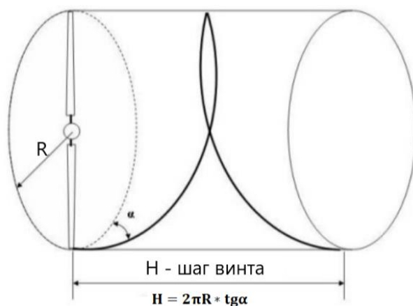
Рис. 65. Шаг винта
