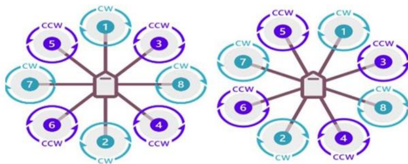
Рис. 56. Схема октокоптера
