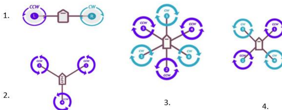
Рисунок 2. Виды схем мультикоптеров.
