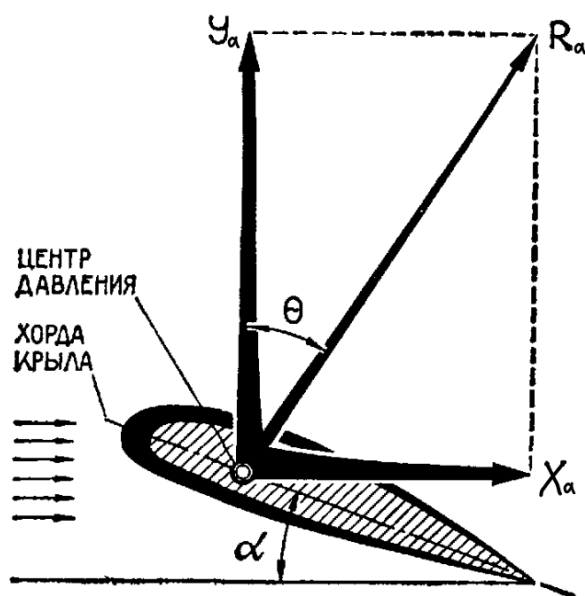
Рис. 44. Составляющие полной аэродинамической силы крыла
